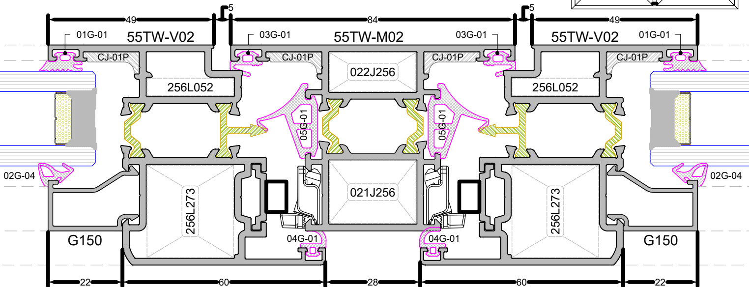
DETAY - 2a DETAIL - 2a
