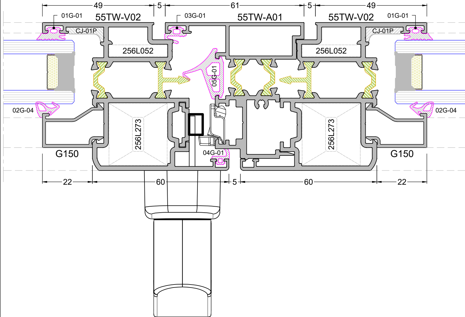
DETAY - 2b DETAIL - 2b
